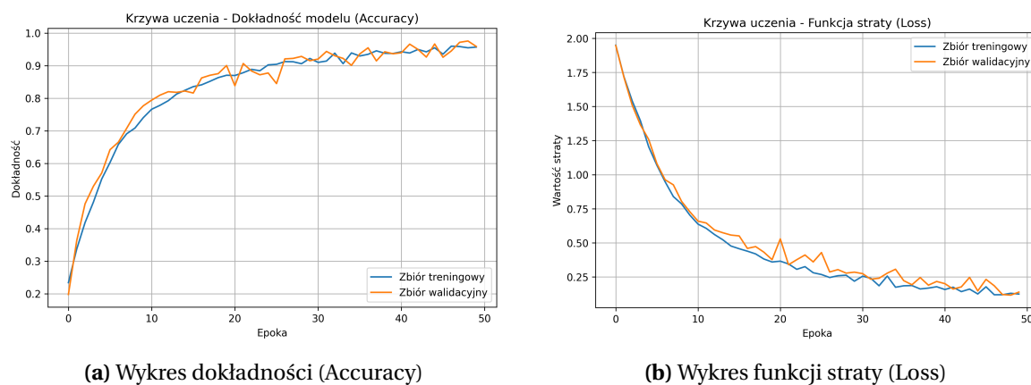
Rysunek 5.1. Krzywe uczenia modelu spłotowego dla zbioru treningowego i walidacyjnego.
