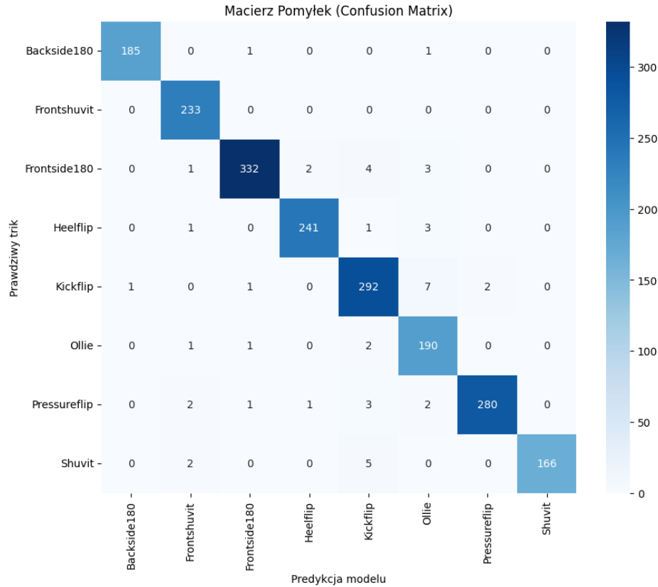
Rysunek 5.2. Macierz pomyłek klasyfikatora na zbiorze testowym.
